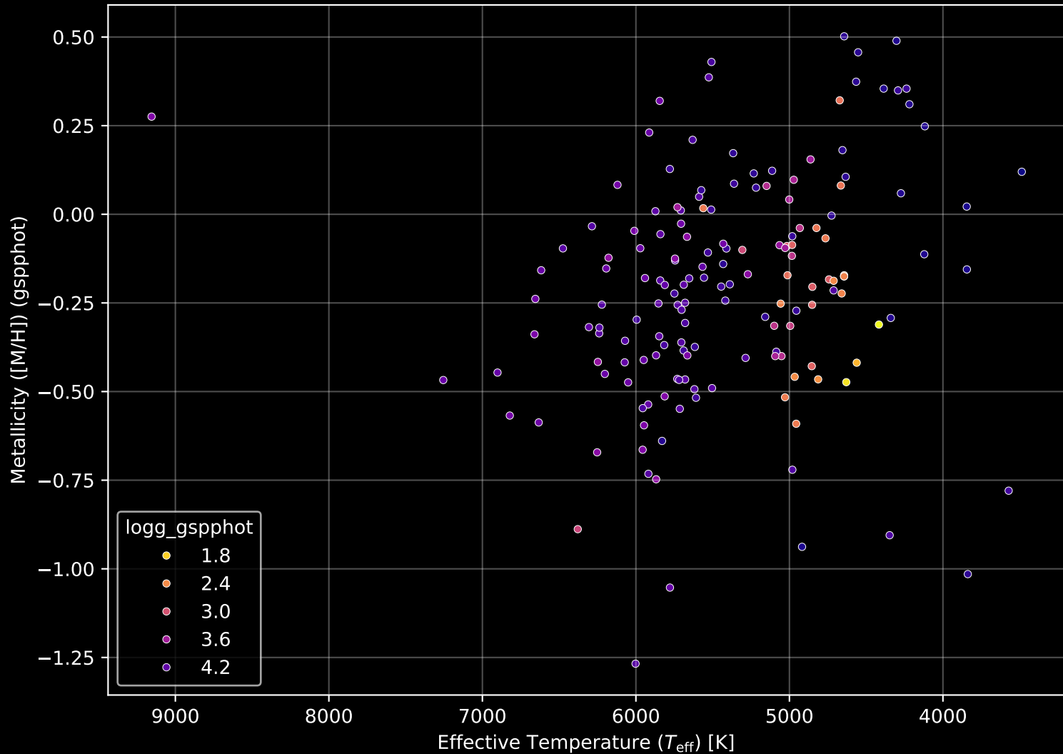
APOGEE DR17 Field: [063+41_MGA] Stellar Population Parameters (n= 162)
